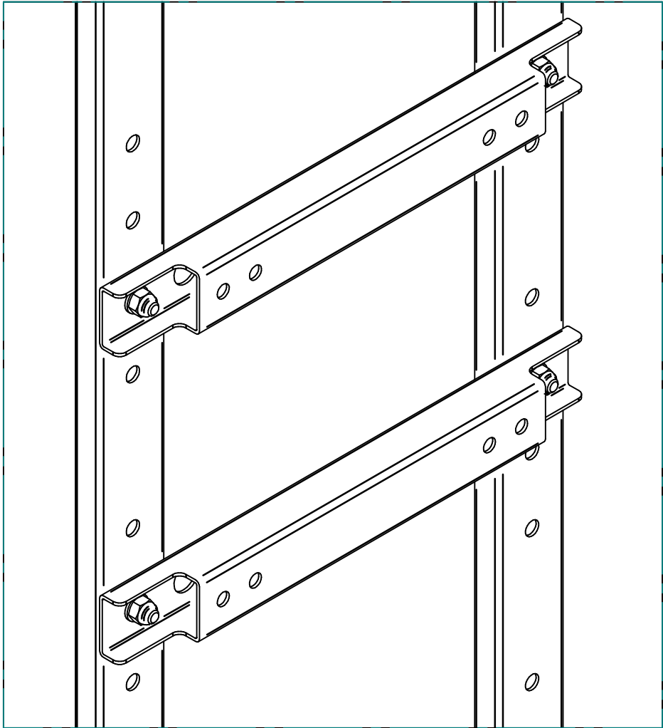
DETTAGLIO B
