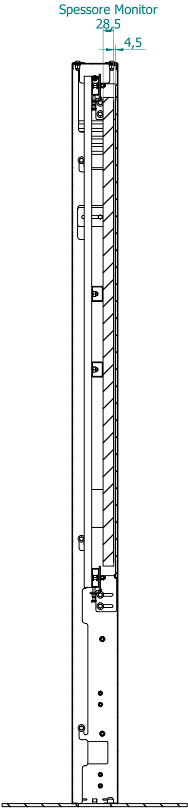
SEZIONE A-A
