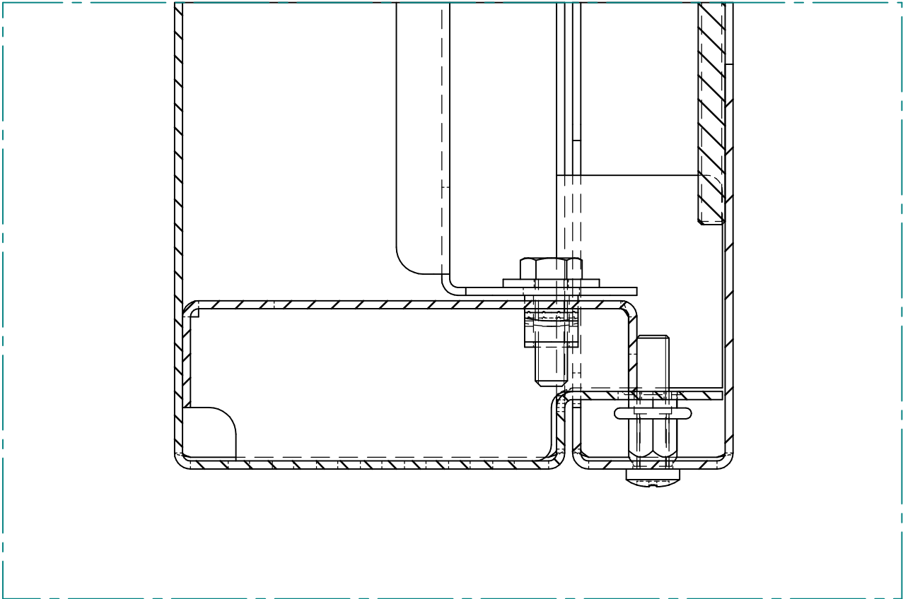
DETTAGLIO C
